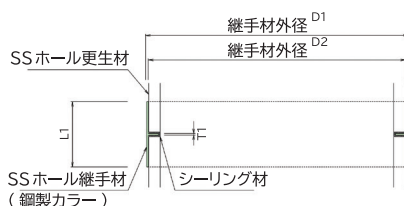
断面図
